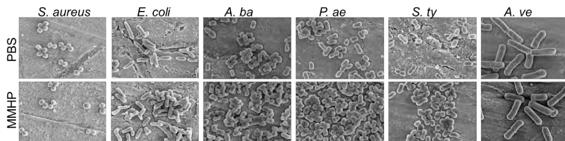
Figure S3. The SEM image of S. aureus , E. coli , A. ba , P. ae , S. ty , and A. ve after antibacterial process.
