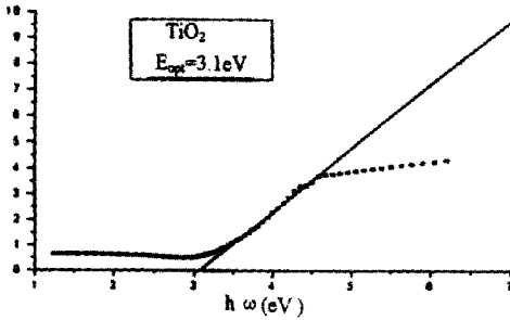
图11 氧缺位TiO 2-x 薄膜的半导体特性
