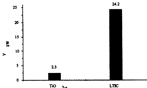
图6 Ti-O薄膜及LTIC与水的界面张力
