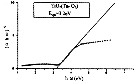
图12 Ta 5+ 掺杂的TiO 2 薄膜的半导体特性
