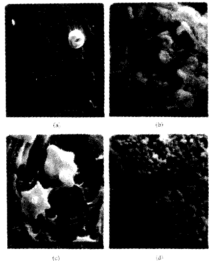
图 9 Ta 5+ 掺杂的 TiO 2 薄膜试片及热解碳的动物体内埋植实验结果(狗心脏内埋植 17 天)
