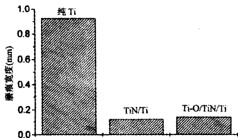
图4 纯钛、TiN薄膜及Ti-O/Ti-N复合薄膜表面划痕宽度
