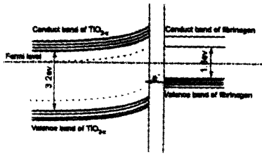
图10 TiO 2-x /纤维蛋白原溶液体系能带结构模型
