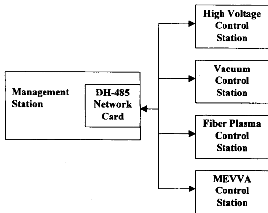
FIG. 1. Schematic of PIIDCS.
